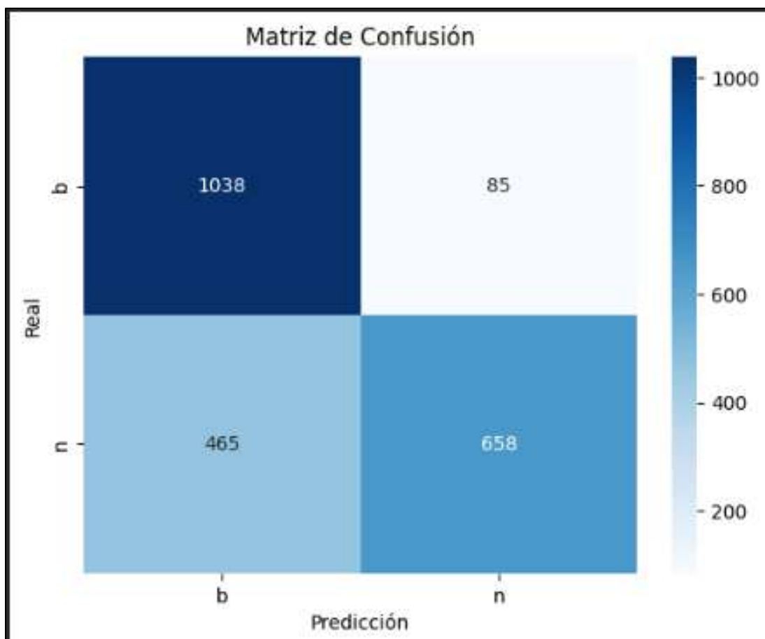
Ilustración 38 Matriz de confusión de MobileNetV2 segunda iteración.
