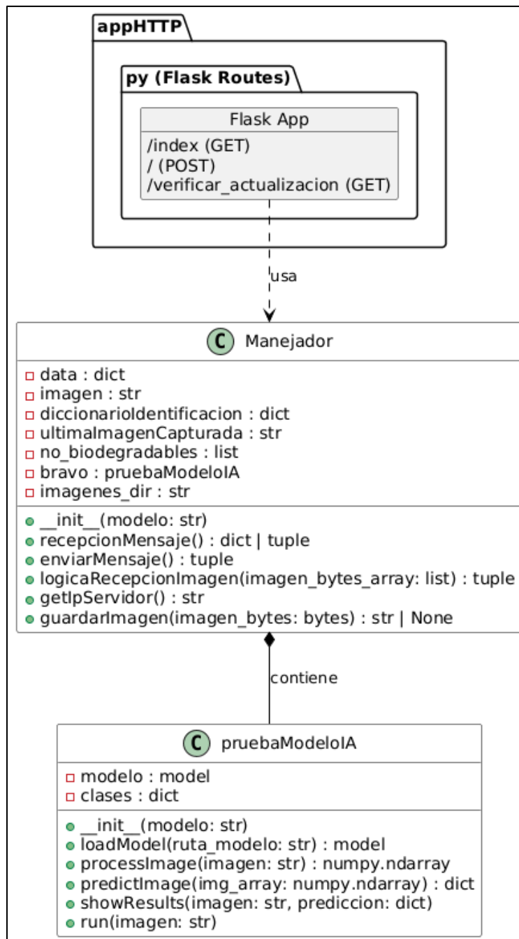
Ilustración 11 Diagrama de clases Python.
