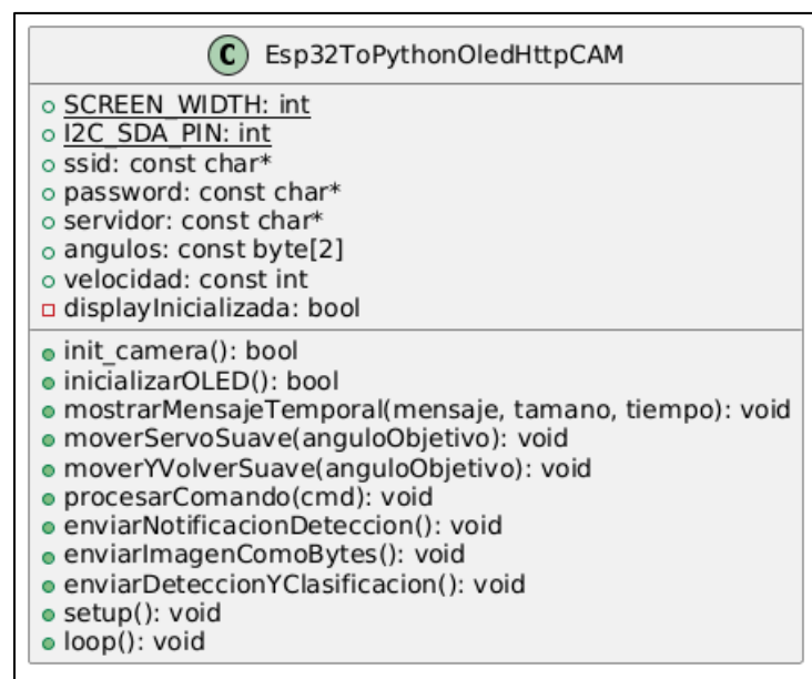
Ilustración 7 Diagrama de clases esp32.
