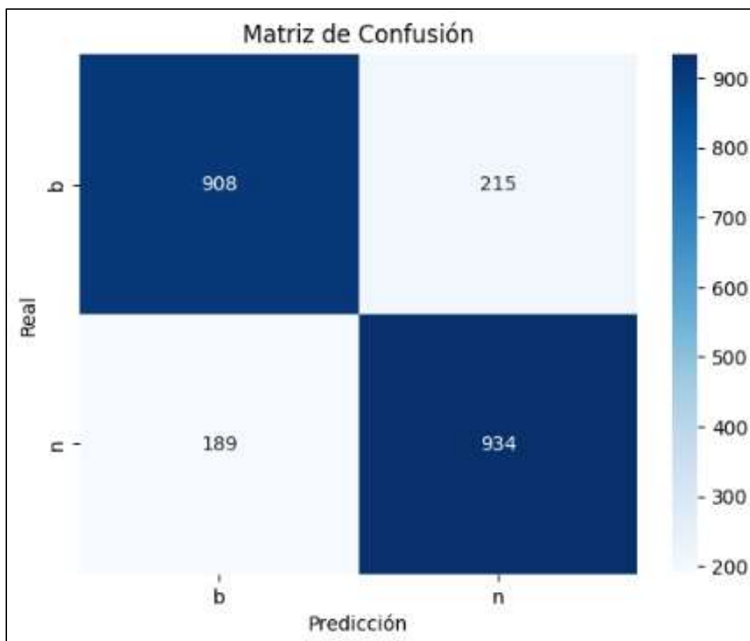
Ilustración 41 Matriz de confusión de MobileNetV2 tercera iteración.
