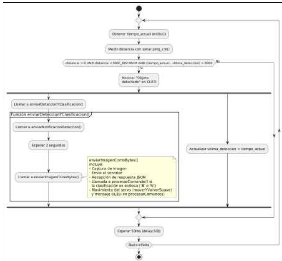
Ilustración 9 Diagrama de flujo del loop esp32.
