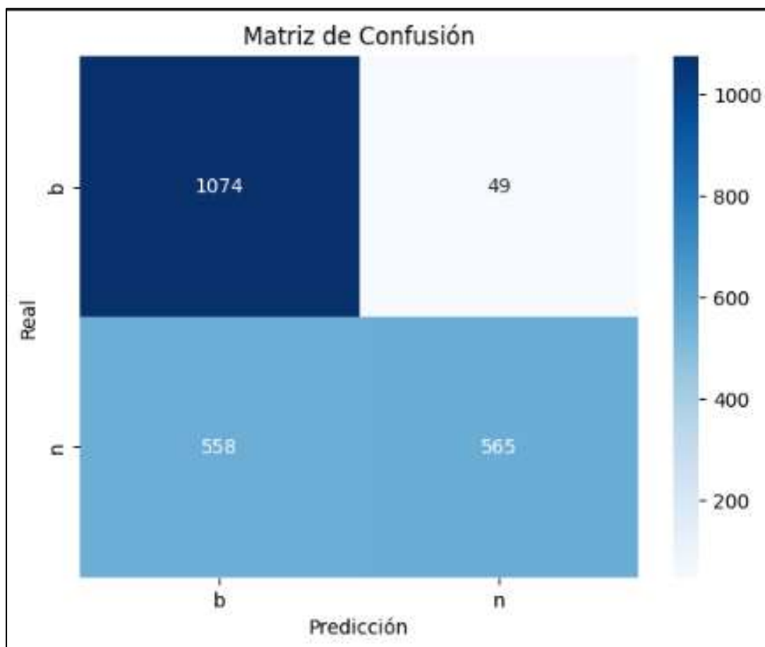
Ilustración 35 Matriz de confusión de MobileNetV2 primera iteración.
