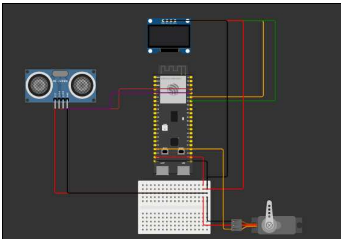
Ilustración 17 Diagrama de electrónico.
