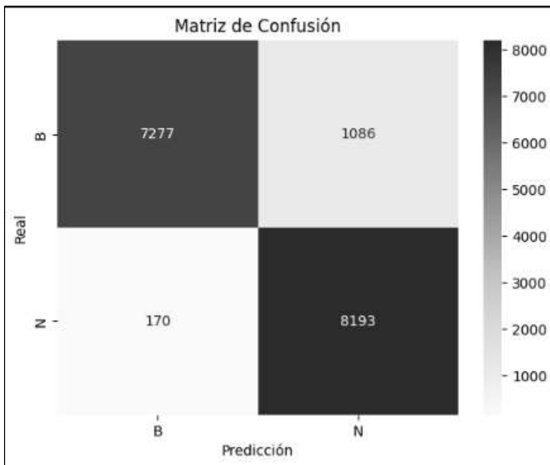
Ilustración 32 Matriz de confusión de ResNet50.
