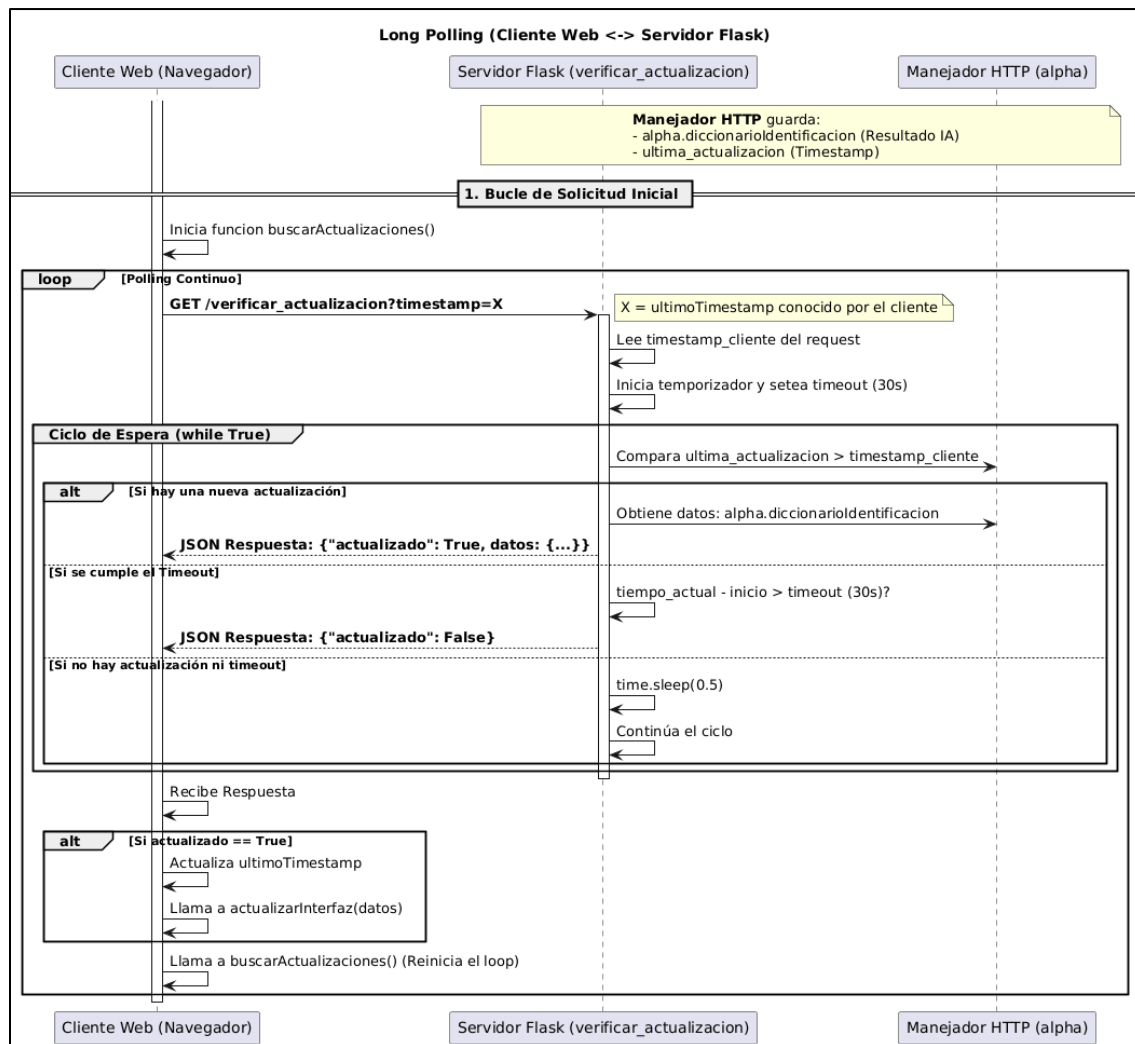
Ilustración 10 Diagrama secuencia Long Polling.
