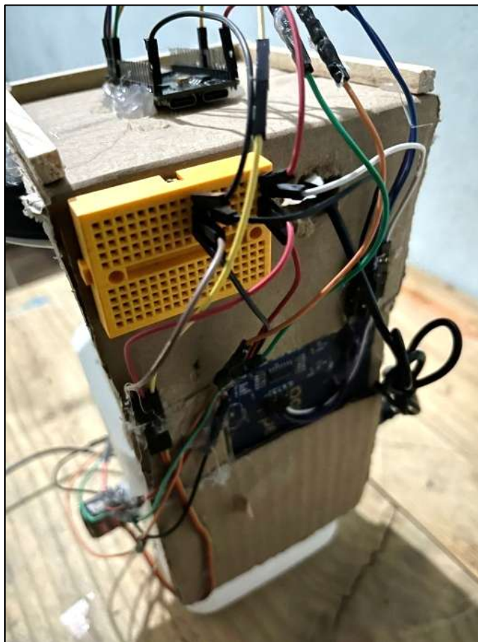
Ilustración 20 Cableado y protoboard prototipo.
