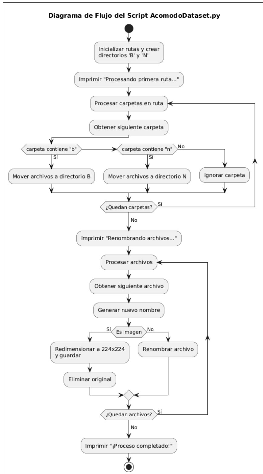
Ilustración 12 Diagrama de flujo AcomodoDataset.
