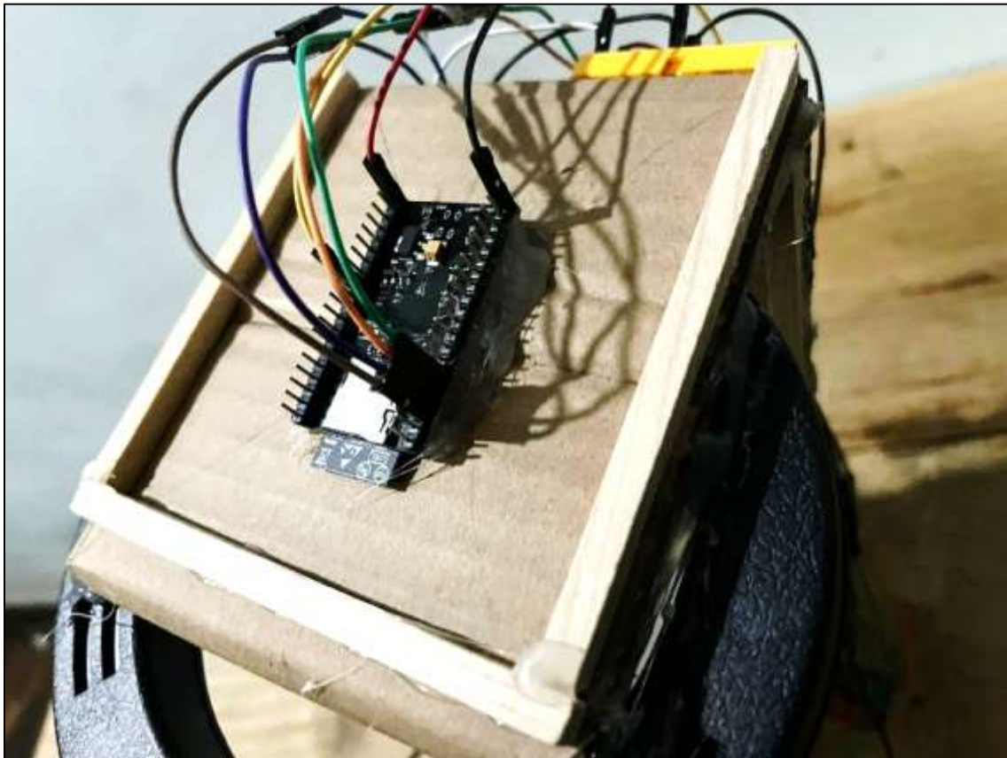
Ilustración 18 ESP32 S3 Cam ubicación.
