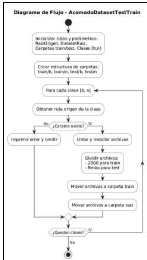
Ilustración 13 Diagrama de flujo AcomodoDatasetTestTrain.
